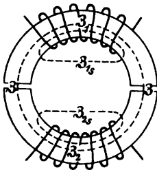
Abb. 194a. Schematische Darstellung der Scheitelwerte der Feldkomponenten.
